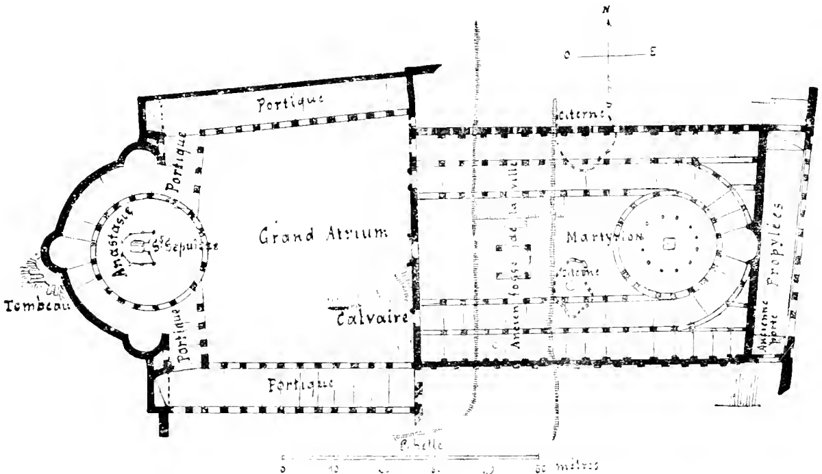
Saint-Sépulcre à Jérusalem construit par sainte Helène vers 310. Plan de la basilique de Constantin, d'après M. SCHICK.
